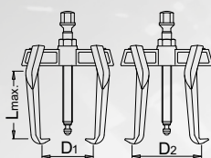
ART. 683/2 Estrattore con due becchi scorrevoli reversibili
